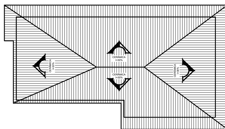
Planta de Cobertura _____ Esc.: 1/150
