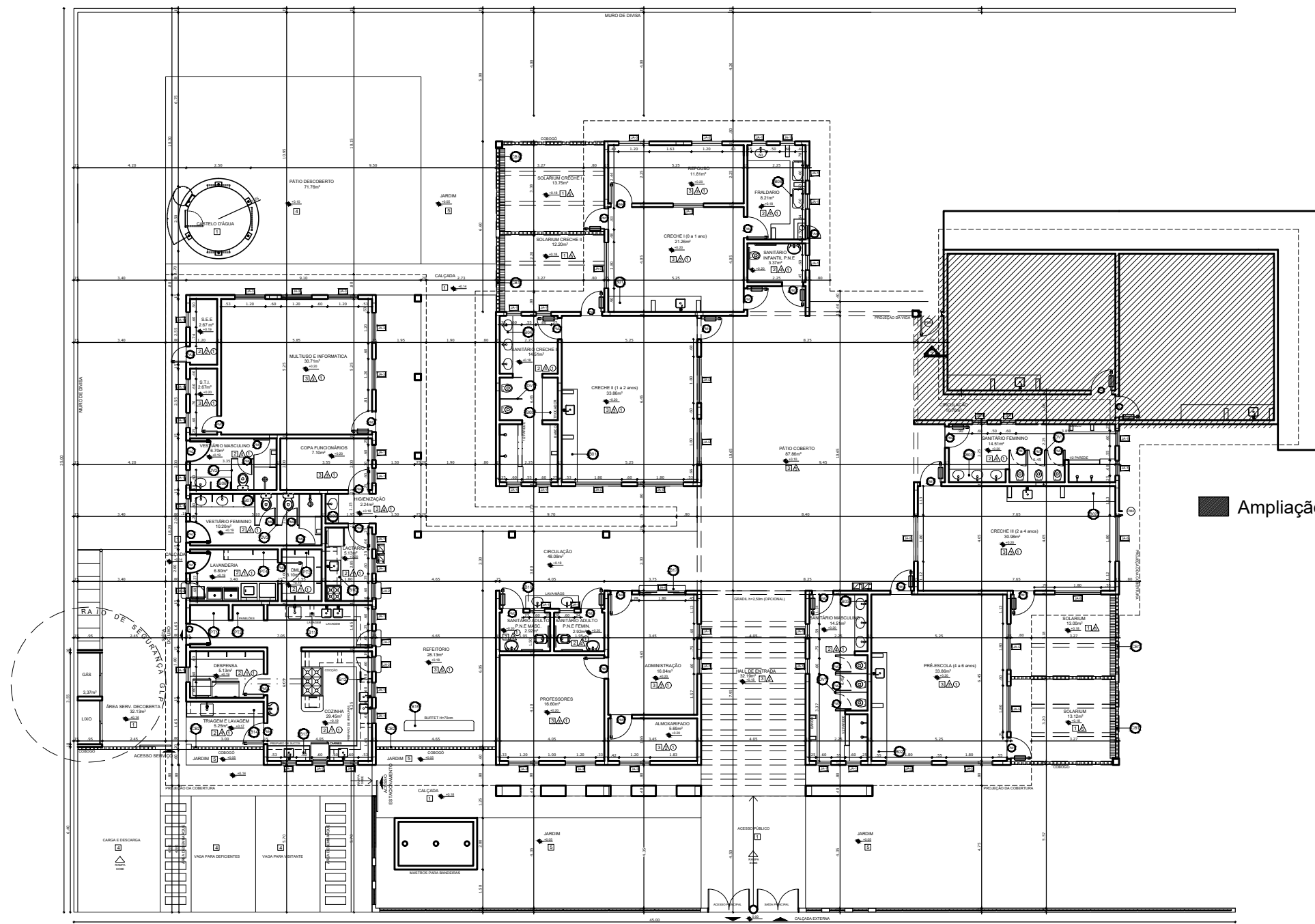
Planta Baixa Creche _____ Esc.: 1/200
